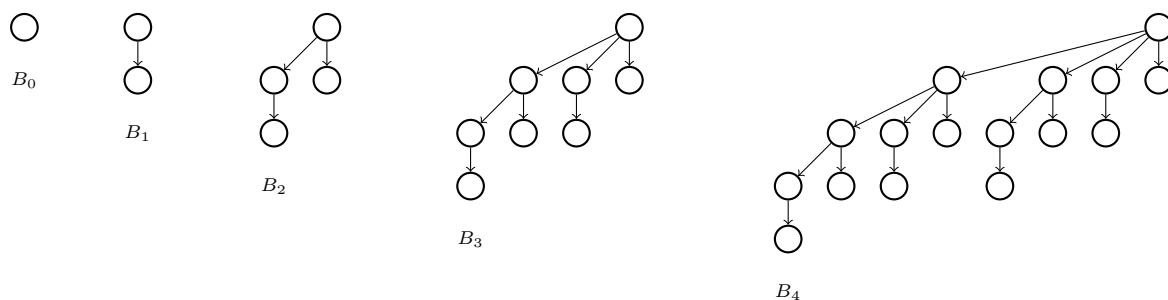
FIGURE 1 – Arbres binomiaux.
